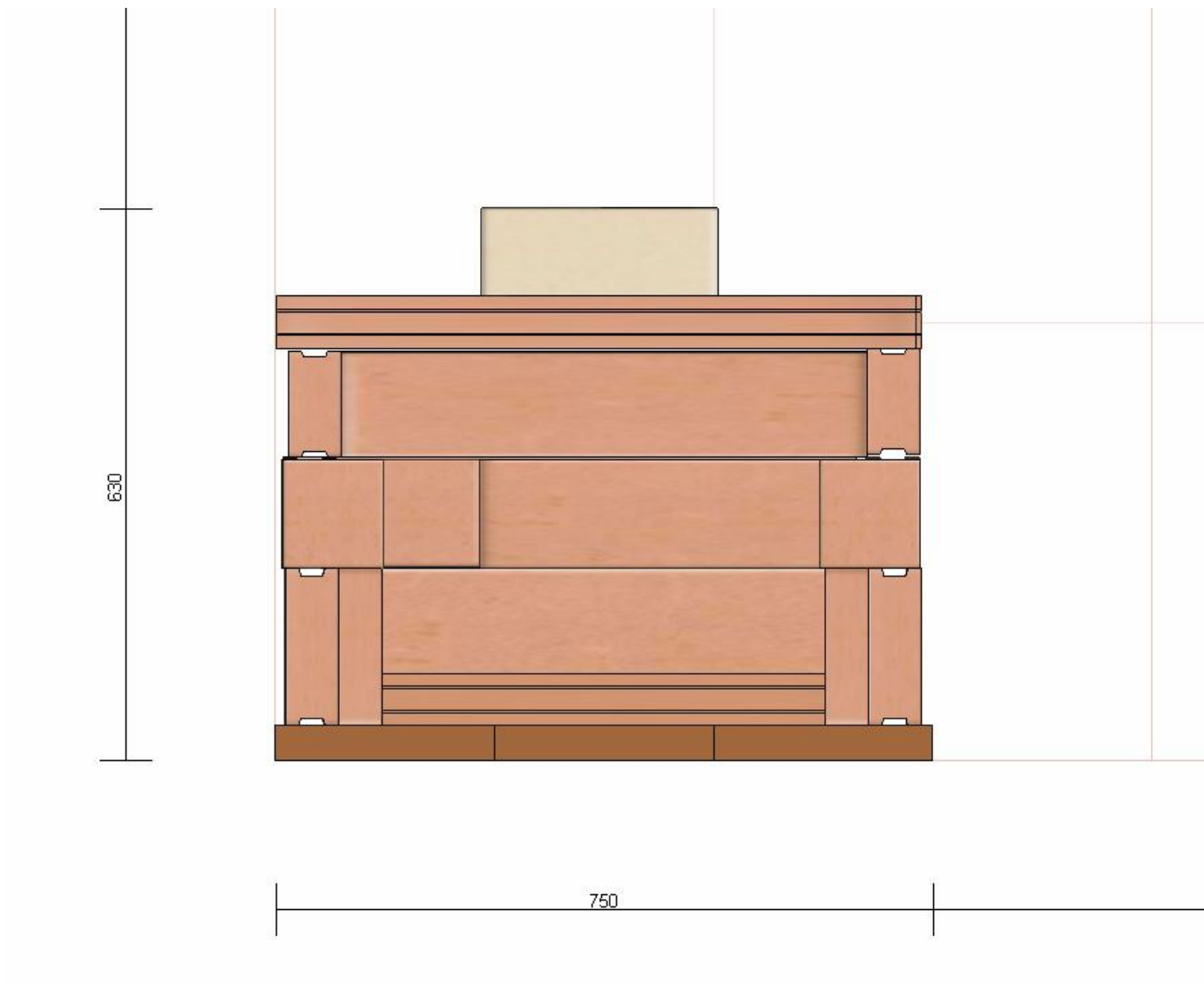
Печь пекарная REMUS 60120R 600x1200 мм вид спереди
