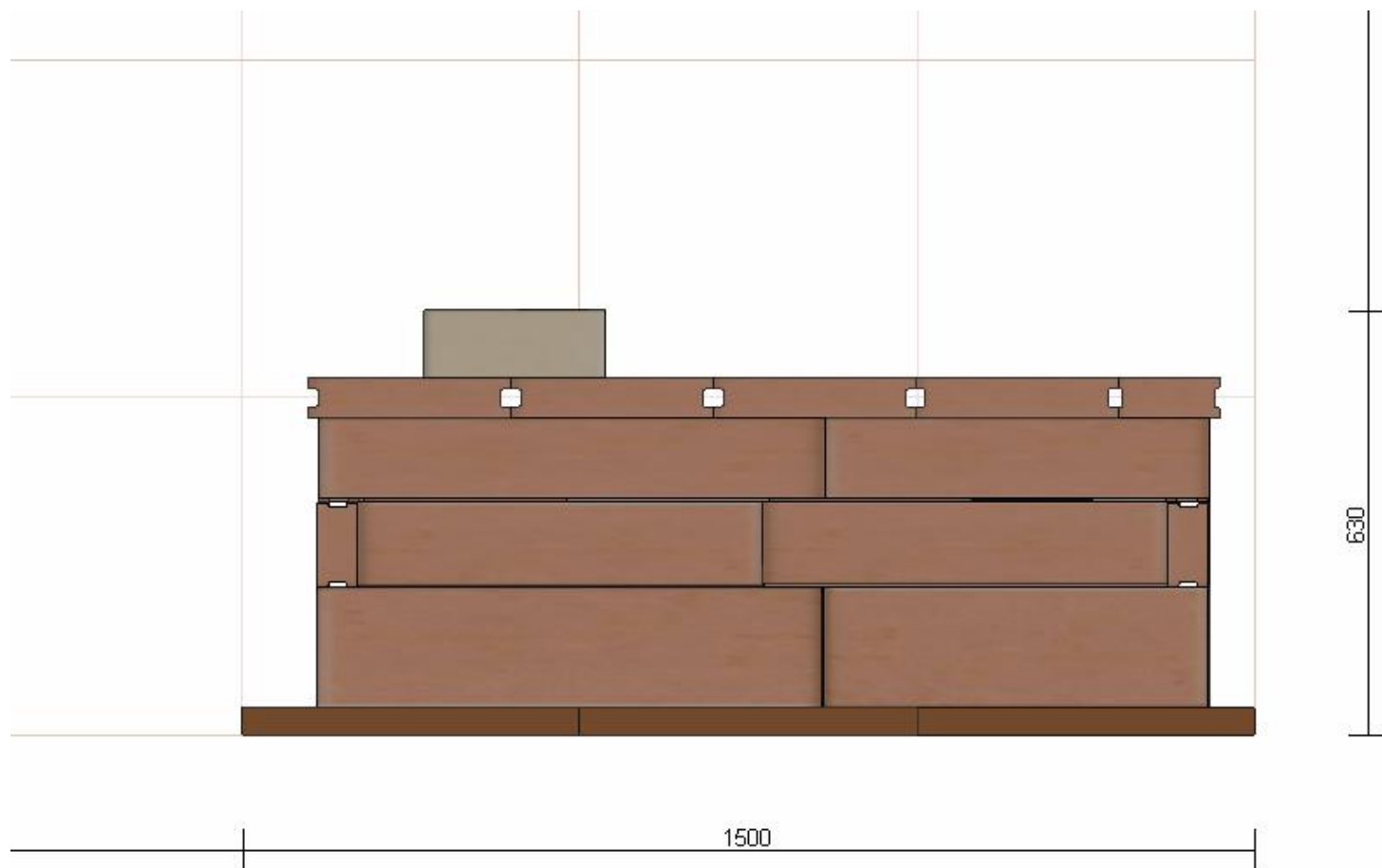
Печь пекарная REMUS 60120R 600x1200 мм вид сбоку
